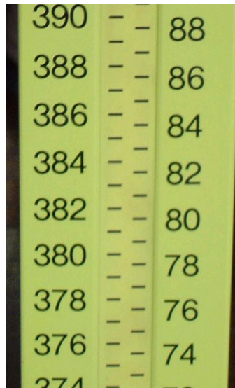
Figura 6.5 – Detalhe de uma mira de ínvar
