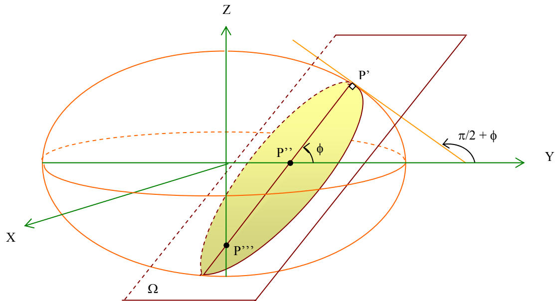
Figura 1.16 – Seção normal primeiro vertical
