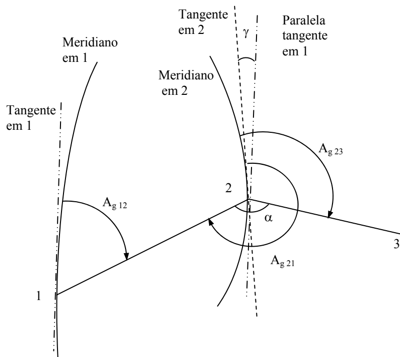
Figura 4.9 – Cálculo do azimuth de uma direção a partir do contra-azimute da direção anterior
