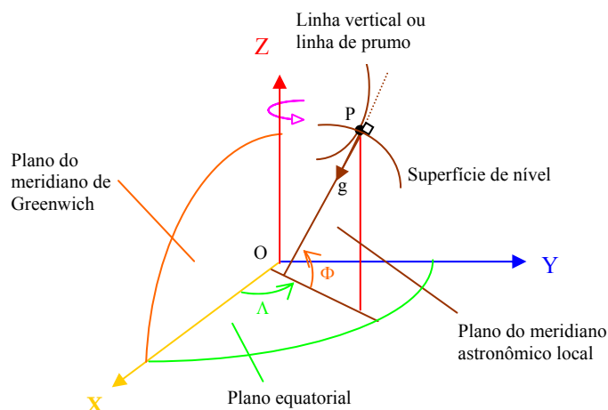
Figura 1.30 – Coordenadas Astronômicas
