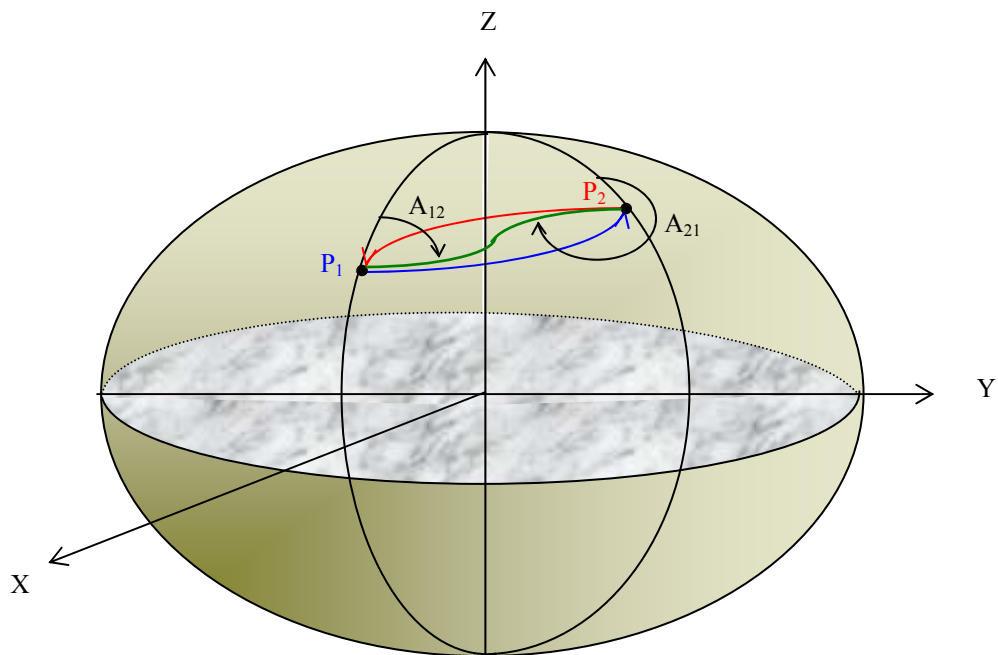
Figura 1.24 - Geodésica
