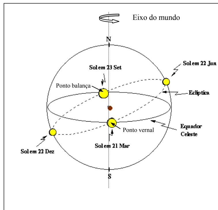
Figura 2.1 – Esfera Celeste
